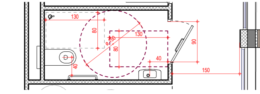
2 DETAIL SANITAIRE PMR Echelle : 1 : 50
