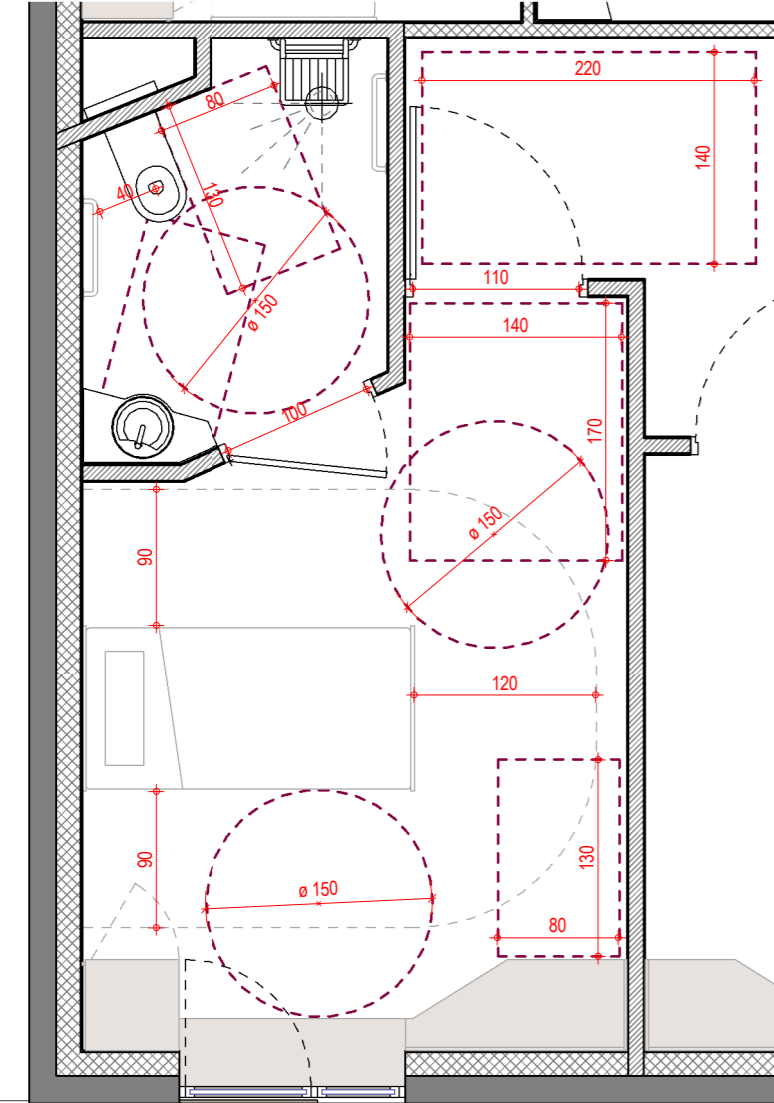
1 DETAIL CHAMBRE PMR Echelle : 1 : 50
